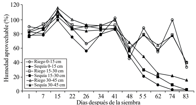
Figura 1. Humedad aprovechable del suelo durante el desarrollo del cultivo de frijol, en ensayos de riego sequía.
