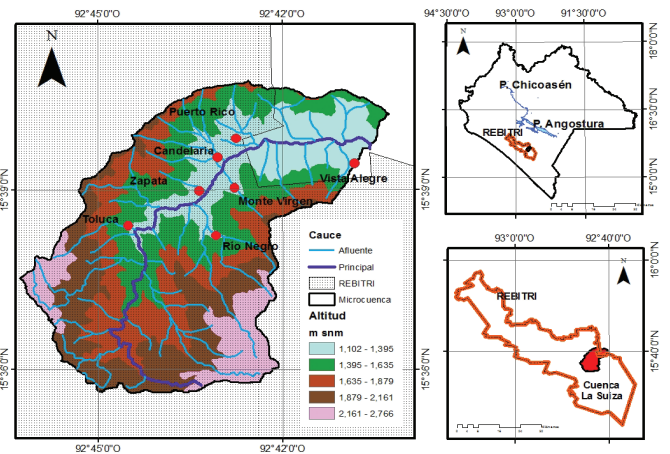
Figura 2. Ubicación de la microcuenca La Suiza. Figure 2. Location of the La Suiza micro watershed.
