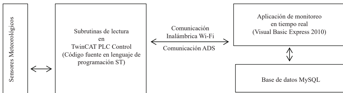
Figura 5. Diagrama del flujo de información. Figure 5. Diagram of information flow.
