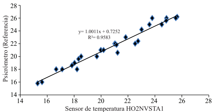
Figura 6. Relación entre en la temperatura de sensor (H02NVST1) y el termómetro seco del psicrómetro.
