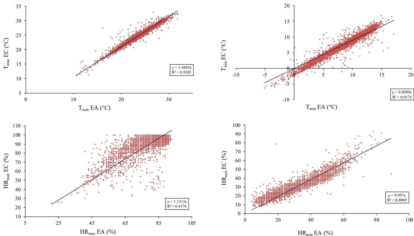
Figura 3. Regresión lineal, con ordenada al origen, entre datos de la EA vs EC para 3a) T_{max} y 3b) T_{min} , y para 3c) HR_{max} y 3d), HR_{min} . Figure 3. Linear regression, with ordinate to the origin, between data from the EA vs EC for 3a) T_{max} and 3b) T_{min} , and for 3c) HR_{max} and 3d), HR_{min} .
