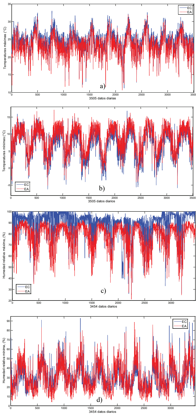
Figura 1. Series de datos de 2004 a 2013 para a) T_{max} , b) T_{min} , c) HR_{Max} , d) HR_{Min} , tanto para estación EA como EC. Figure 1. Data Series from 2004 to 2013 for) T_{max} , b) T_{min} , c) HR_{Max} , d) HR_{Min} , both EA and EC station.
