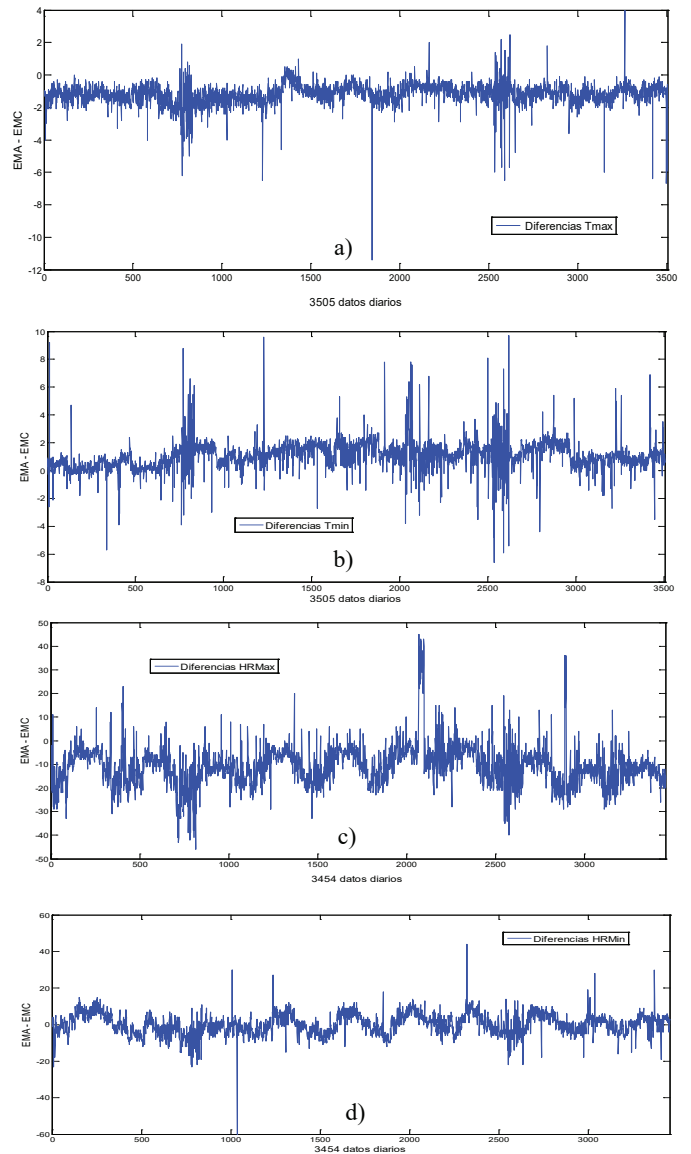
Figura 2. Diferencias de los datos de las variables de ambas estaciones. Figuras 2a) y 2b) diferencias de las variables temperatura máxima y mínima (EA-EC), respectivamente. Figuras 2c) y 2d) diferencias de las variables humedad relativa máxima y mínima (EA-EC), respectivamente.
