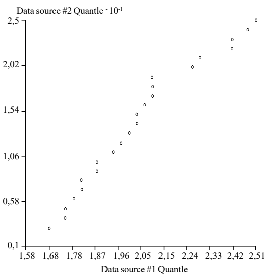
Figura 4. Probabilidad normal para la variable lámina total (mm) y variable rendimiento (kg ha -1 ). Figure 4. Normal probability for variable total sheet (mm) and variable yield (kg ha -1 ).
