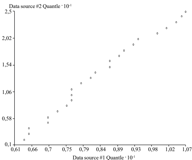
Figura 4. Probabilidad normal para la variable lámina total (mm) y variable rendimiento (kg ha -1 ). Figure 4. Normal probability for variable total sheet (mm) and variable yield (kg ha -1 ).
