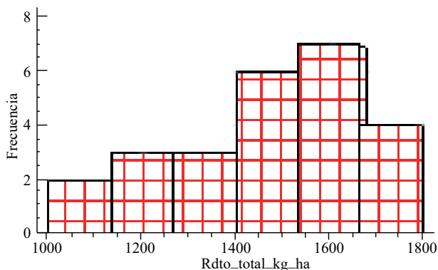
Figura 3. Histograma de frecuencias para el rendimiento (kg h -1 ). Figure 3. Frequencies histogram for yield (kg h -1 ).
